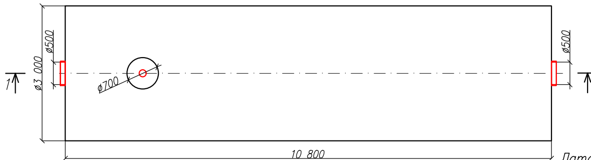
Вид сверху
