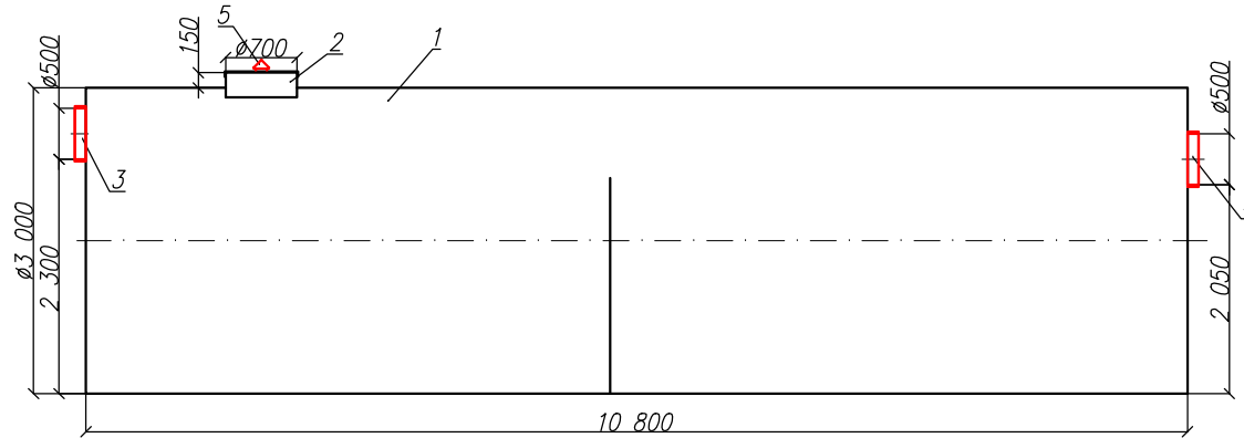
Вид сверху
